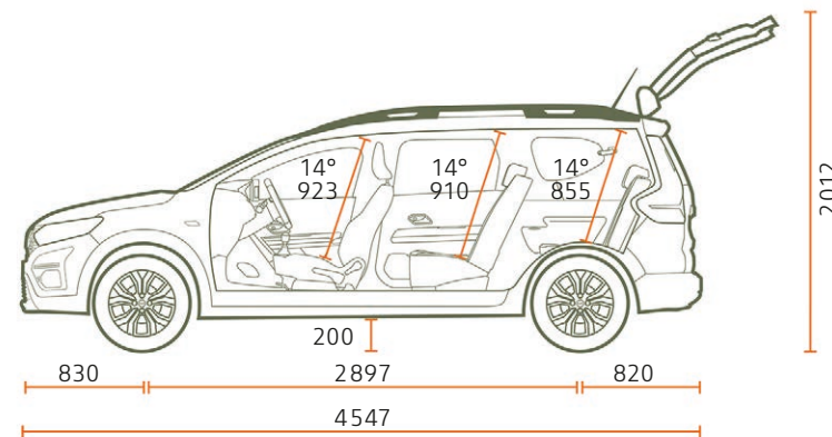
VISTA LATERALE VERSIONE 7 POSTI
